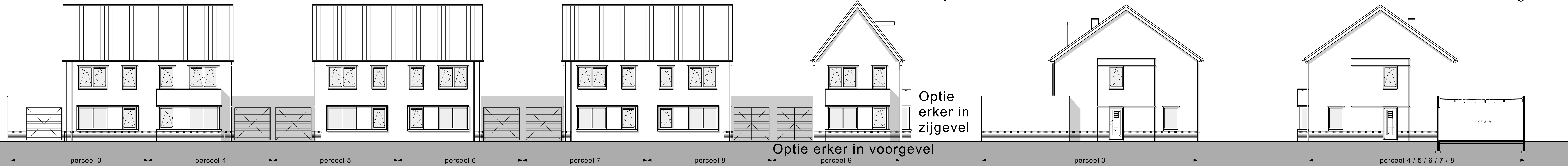
VOORGEVEL (schaal 1 :100)
