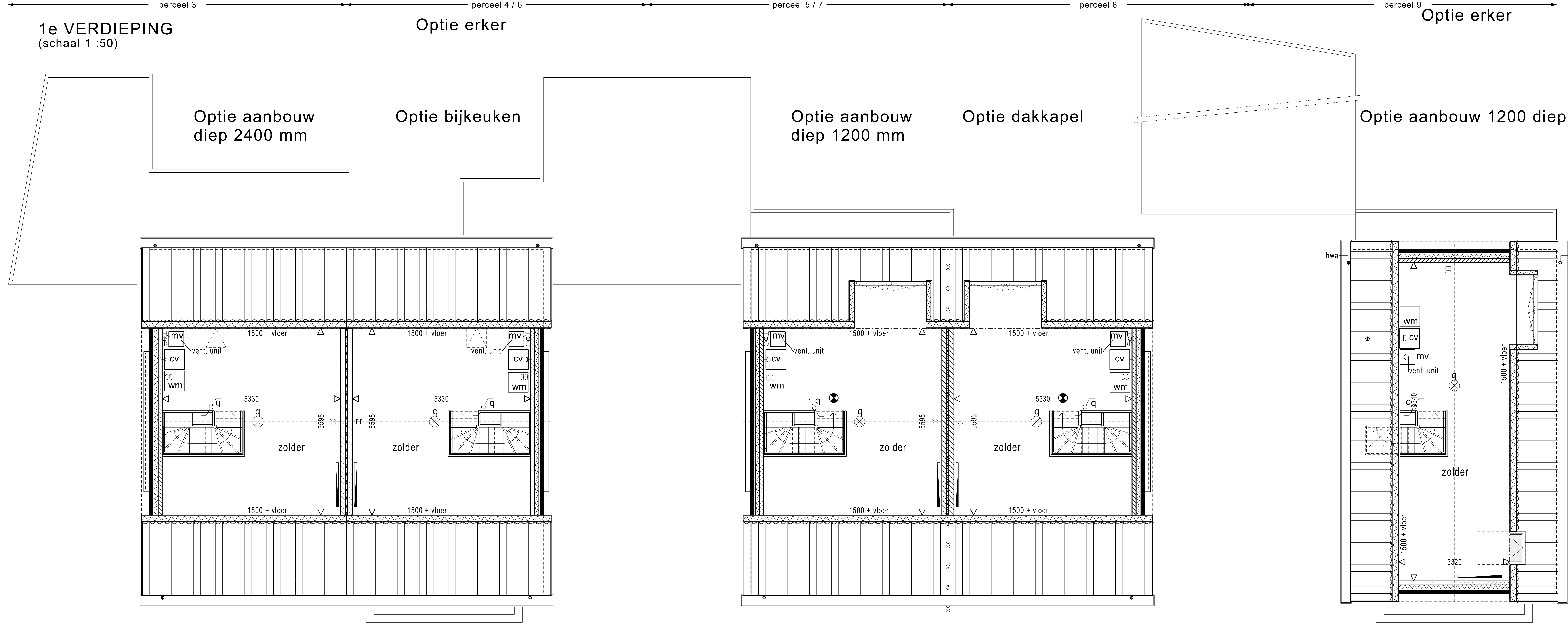
2e VERDIEPING (schaal 1 : 50)
