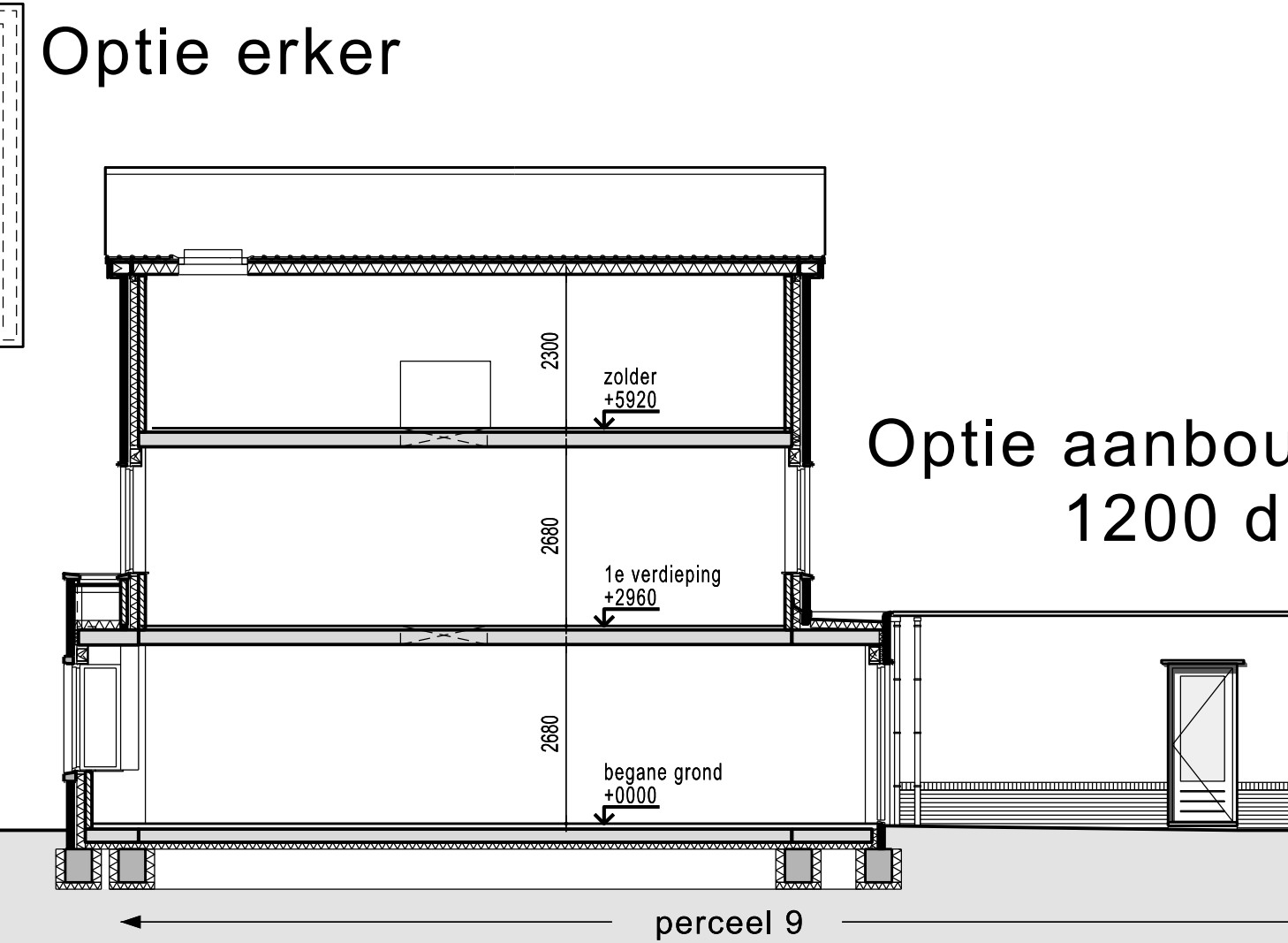
DOORSNEDEN (schaal 1 : 100)
