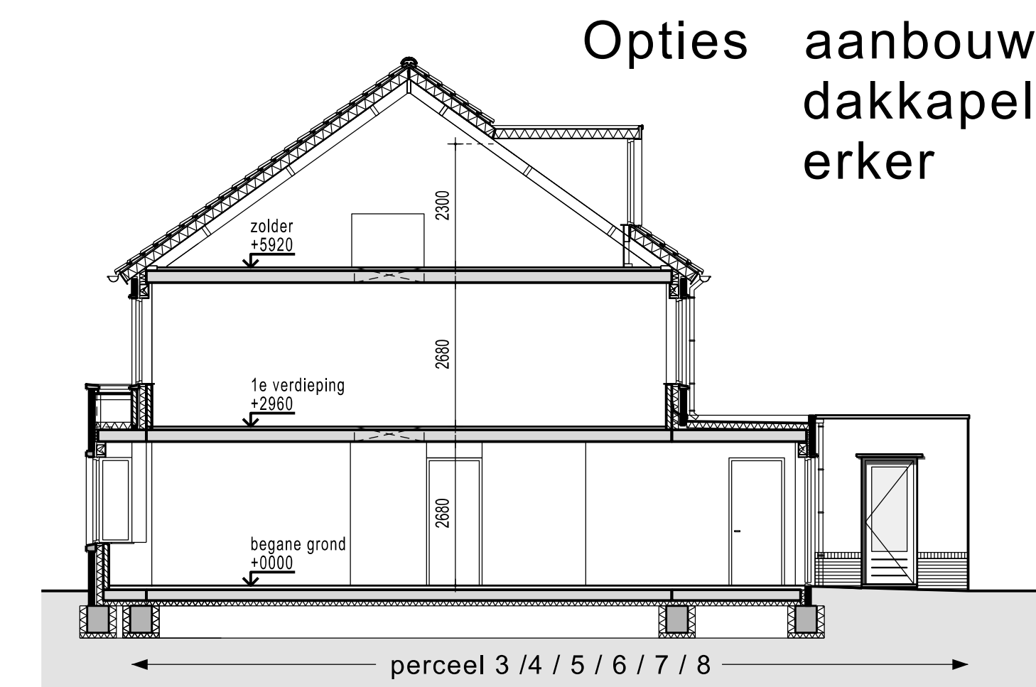
DOORSNEDEN (schaal 1 : 100)
