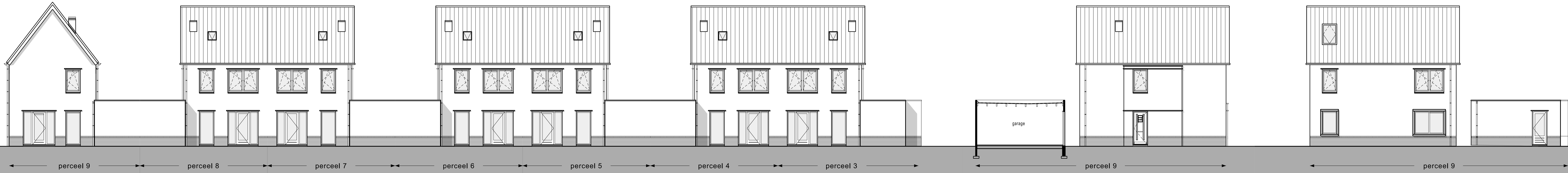
ACHTERGEVEL (schaal 1 :100)
